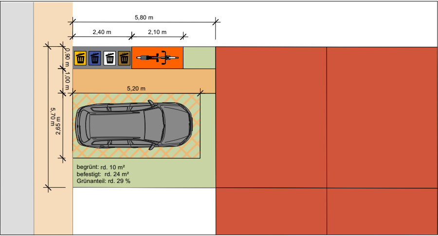
Schritt 3 - Gebäudezuwegung, PKW-Stellplatz, Müllstandort und Fahrrad-Stellplatz
